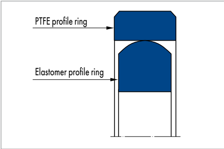
Merkel Omegat OMK-S
