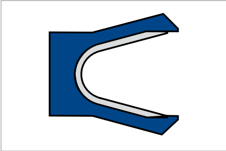
Forseal FOI made of PTFE
