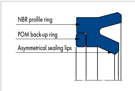
Merkel U-Ring NI 250
