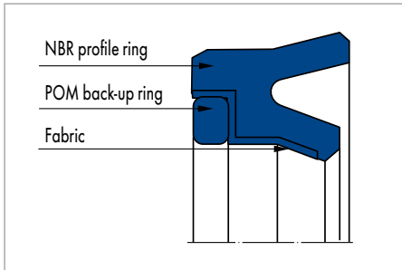
Merkel U-Ring NI 400
