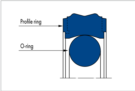
Merkel Omegat OMK-PU
