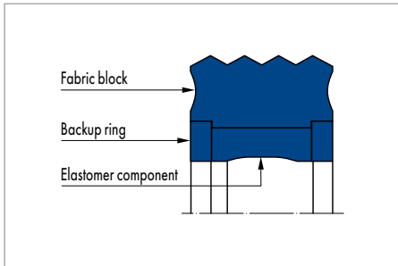
Merkel Rotomatic M 19
