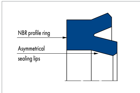
Merkel U-Ring NA 150
