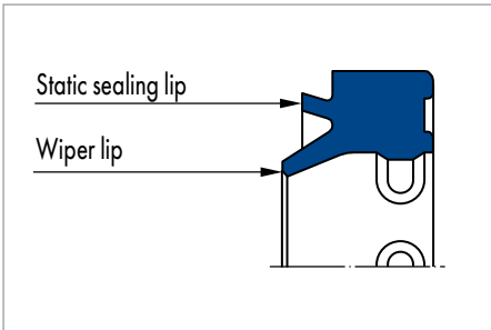
Merkel Wiper PU 5
