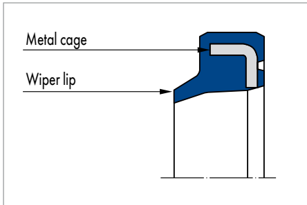
Merkel Wiper PU 7
