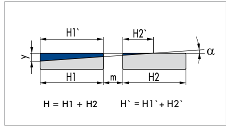
Fig. 11 Usable guide width
