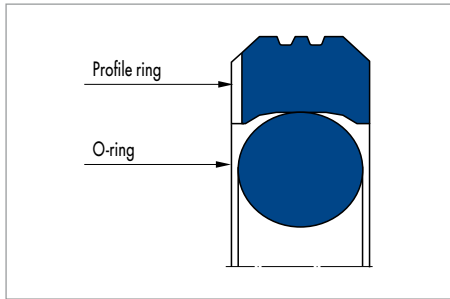
Merkel Rotomatic M 16
