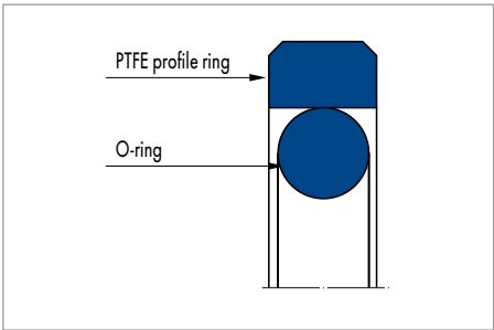
Merkel Omegat OMK-MR
