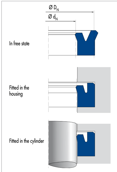
Fig. 2 Rod seal
