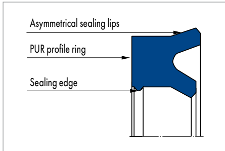
Merkel U-Ring NI 300
