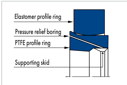
Merkel Omegat OMS-S PR
