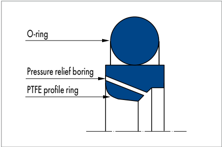
Merkel Omegat OMS-MR PR
