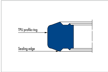
Merkel Stirromatic SRC
