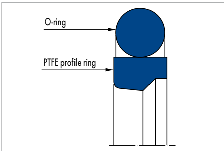
Merkel Omegat OMS-MR
