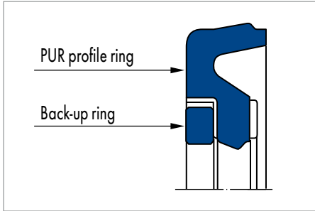
Merkel U-Ring Syprim SM
