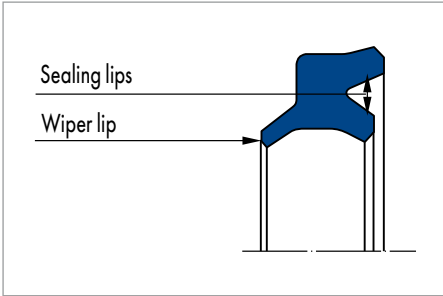
Merkel Double Wiper PU 11
