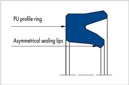
Merkel U-Ring TM 20
