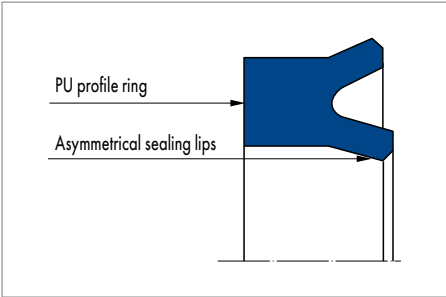
Merkel U-Ring NA 300
