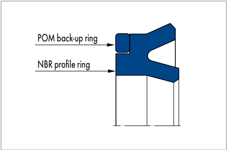
Merkel U-Ring NA 250
