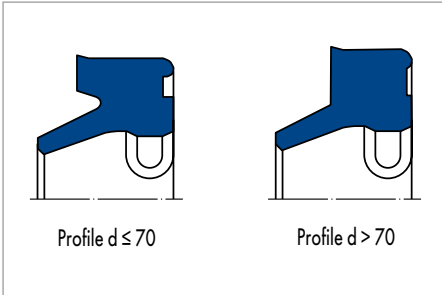
Merkel Wiper PU 6
