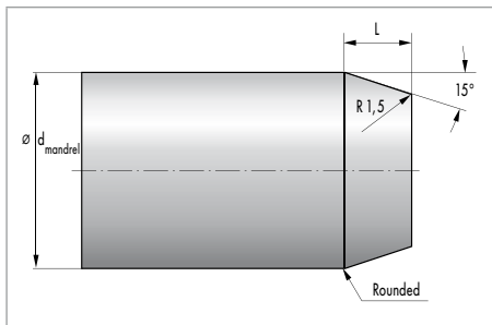
Fig. 50 Calibrating mandrel
